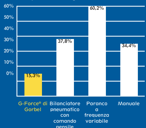
Figura 3: Percentuale dei sollevamenti che superano la soglia della forza
